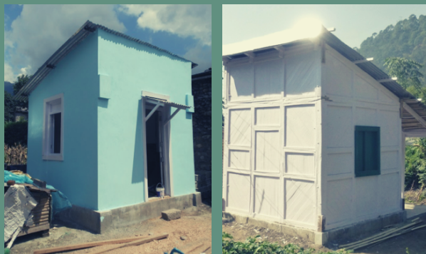
Prototipos antisísmicos Awasuka. Awasuka Antiseismical prototypes.
